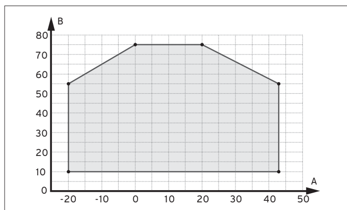
Meze použití, ohřev teplé vody
