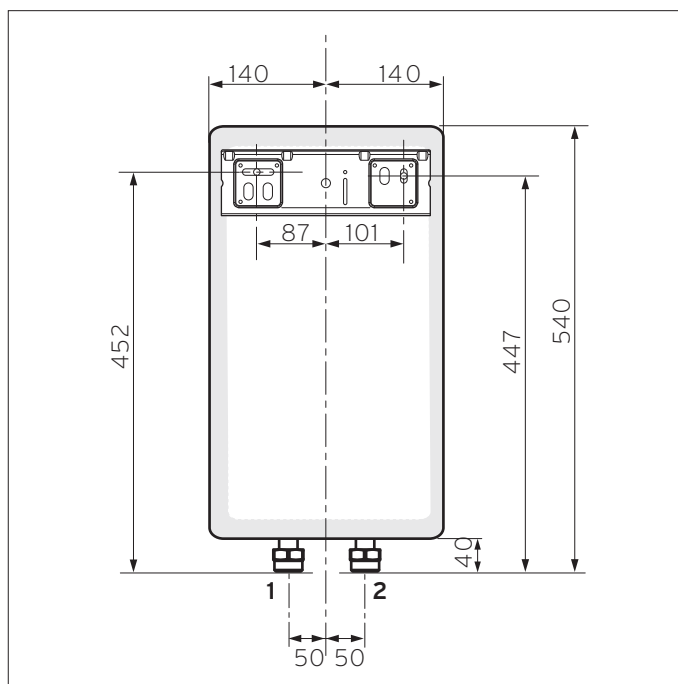
VWZ MEH 60 - přípojky a rozměry
