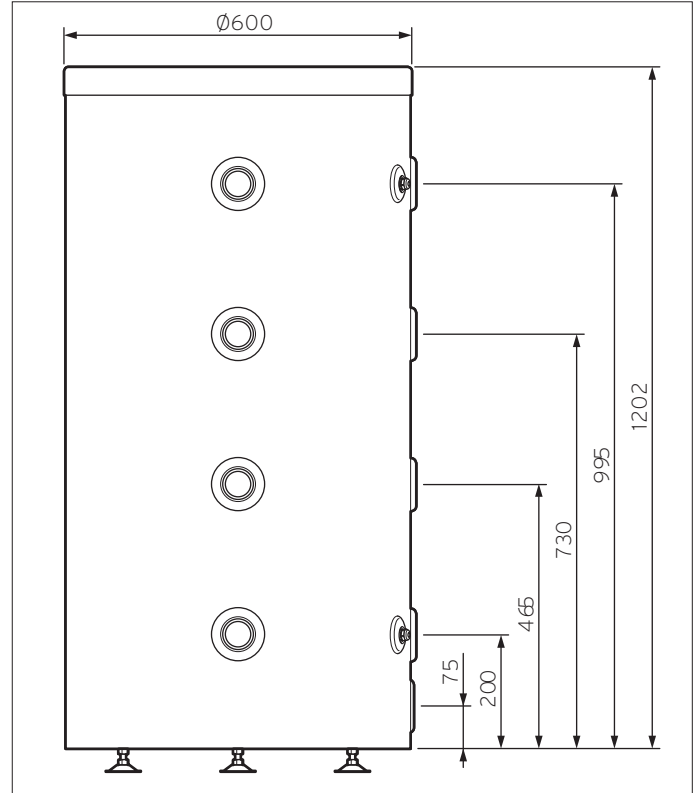
Obr. 611: Rozměry zásobníku
