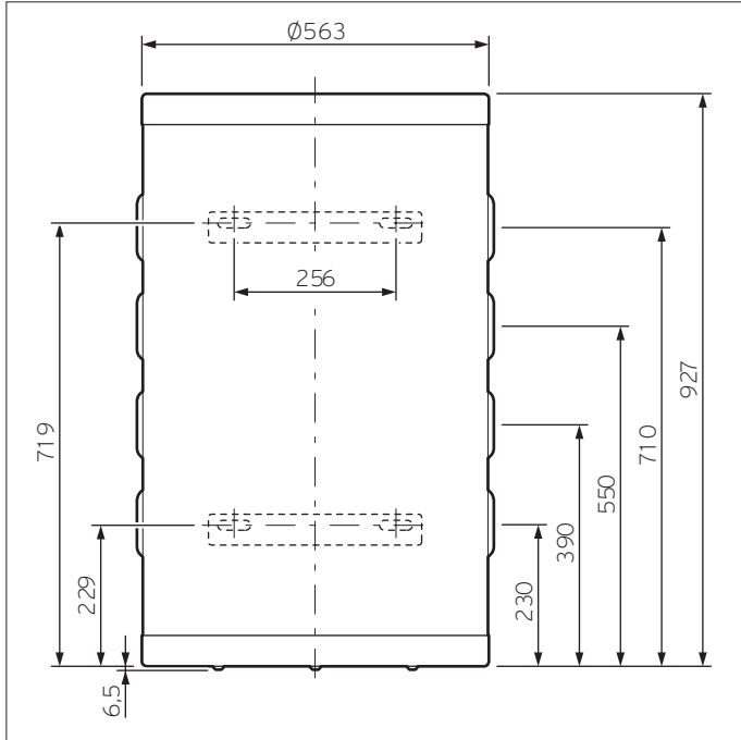
Obr. 610: Rozměry zásobníku
