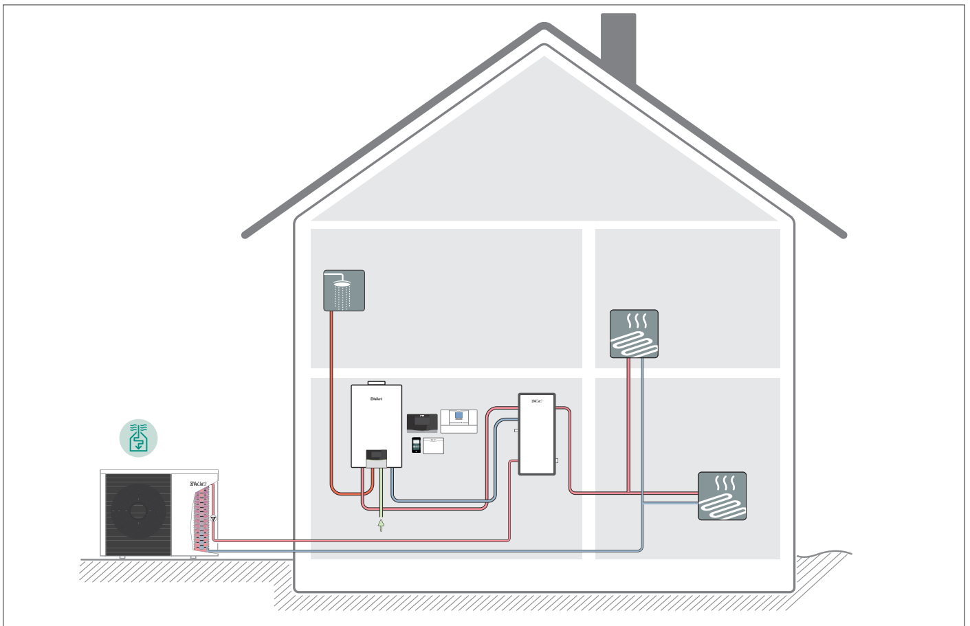
Tepelné čerpadlo aroTHERM plus v bivalentním způsobu provozu - schéma systému
