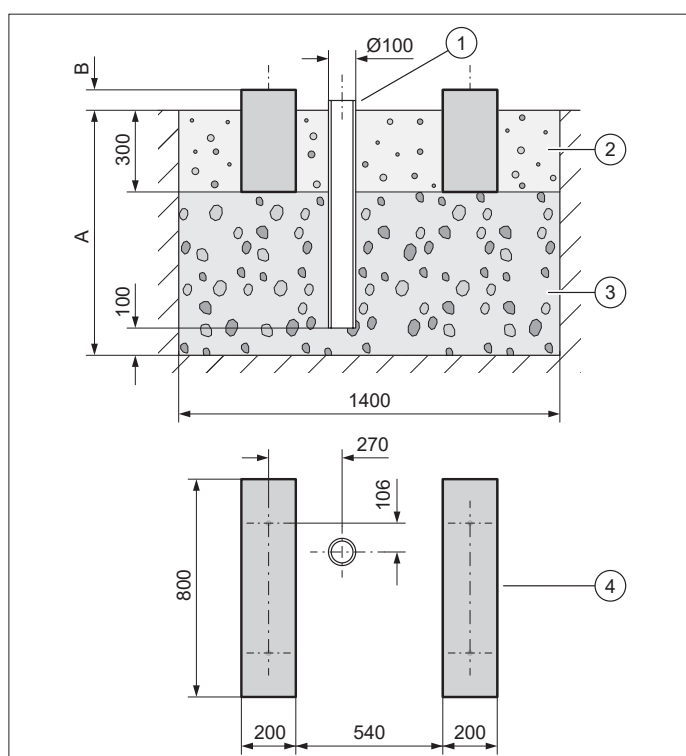
Schéma s rozměry, zhotovení základu
