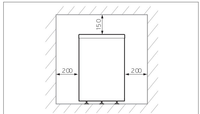
Obr. 612: Minimální odstupy
